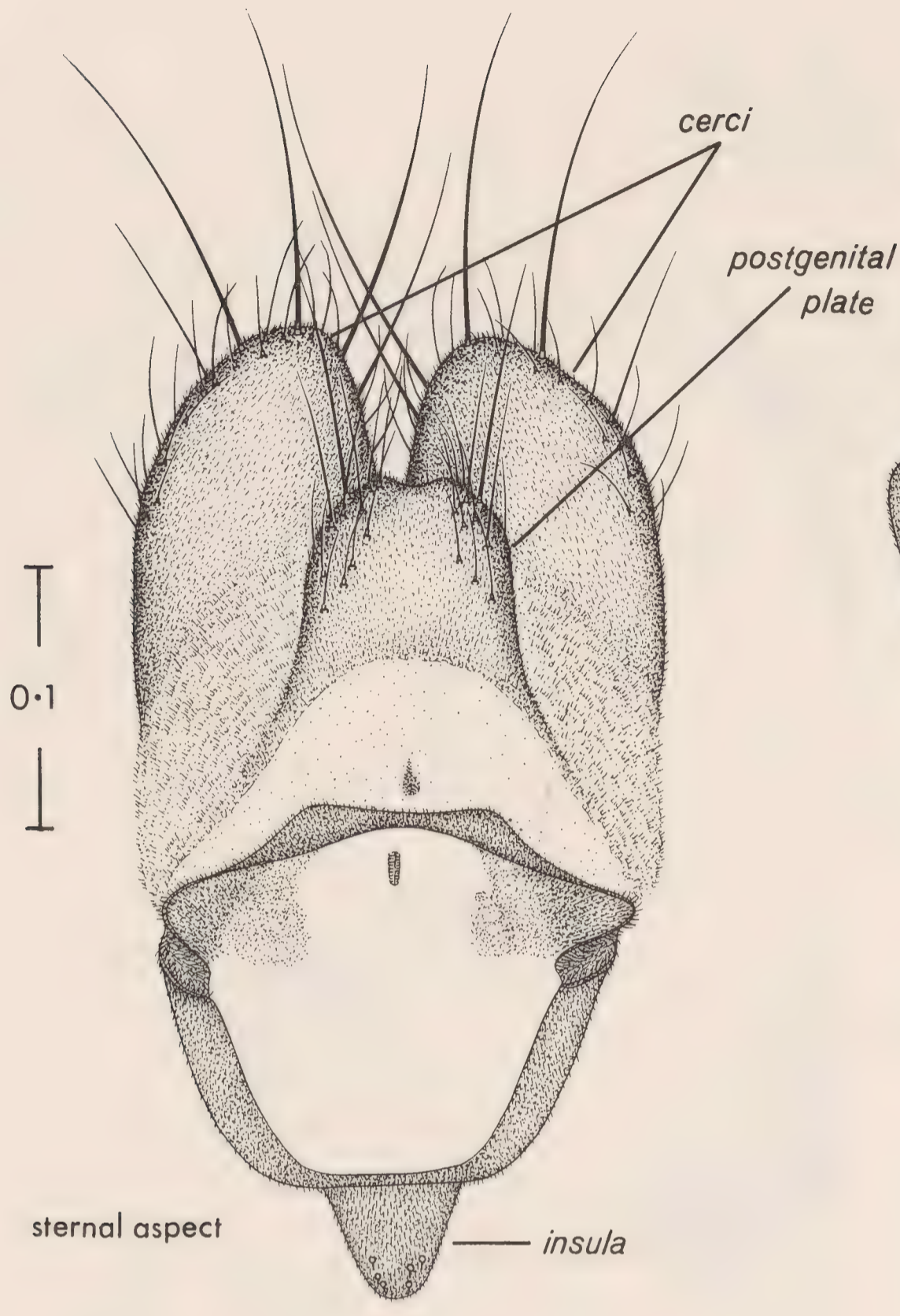
Fig. 12 ♀ terminalia
